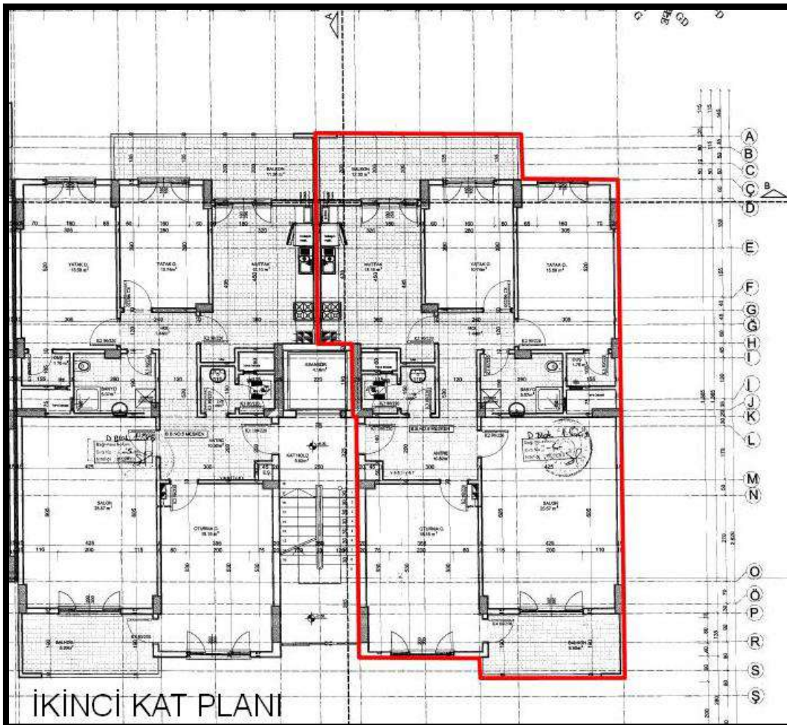
Mimari proje
