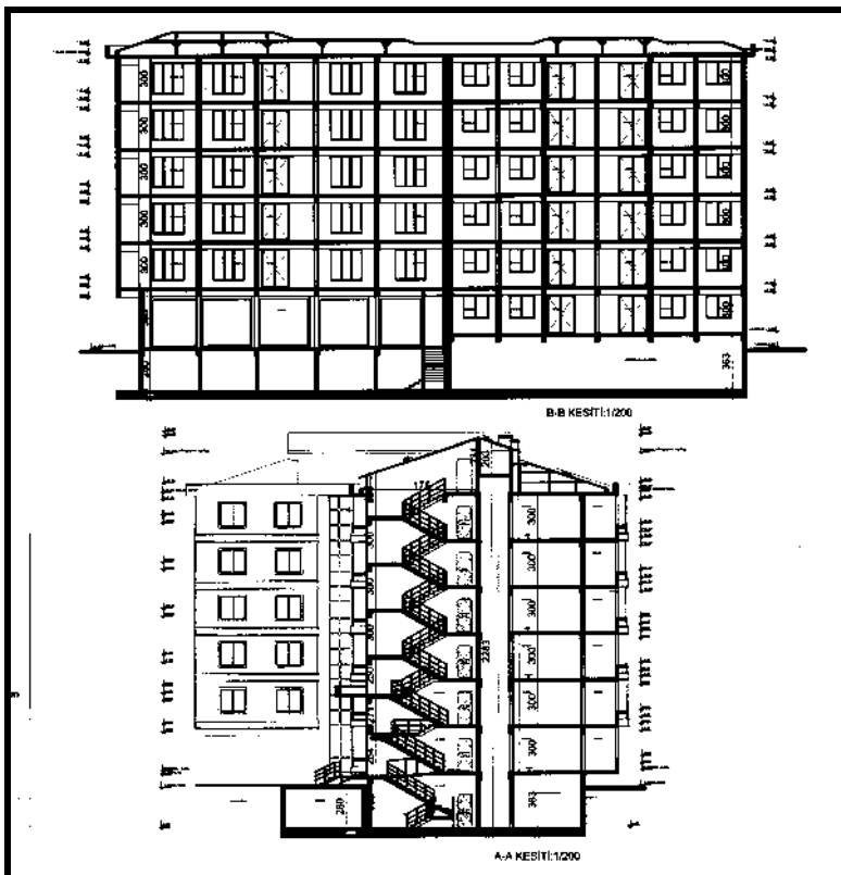
Bina kesiti görünümü
